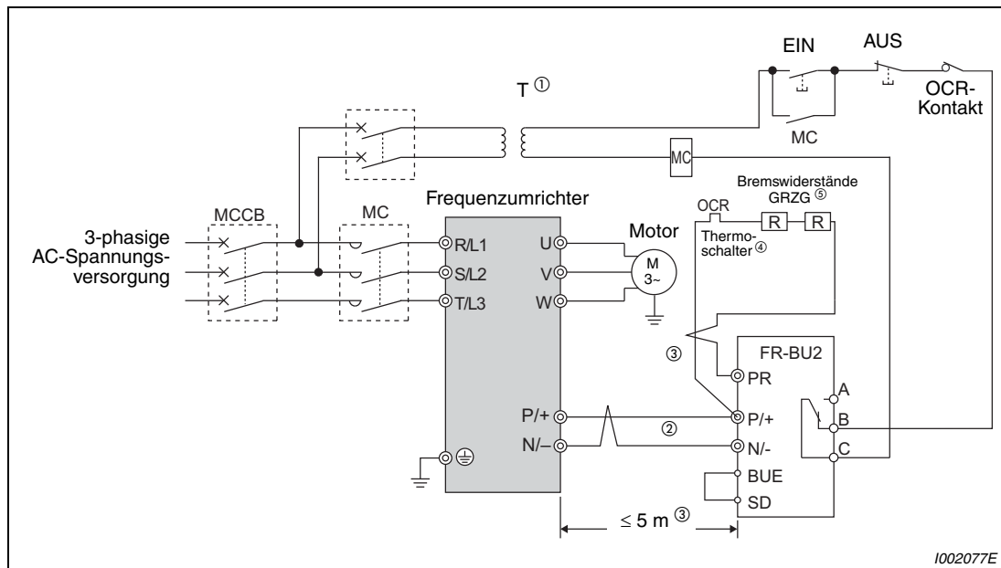
Abb. 3-29: Anschluss der Bremsseinheit vom Typ FR-BU2
