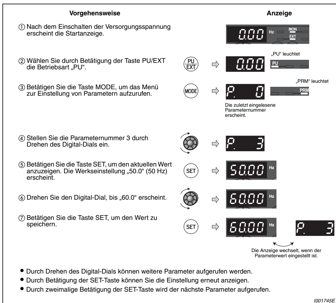
Abb. 5-2: Einstellung der Basisfrequenz
