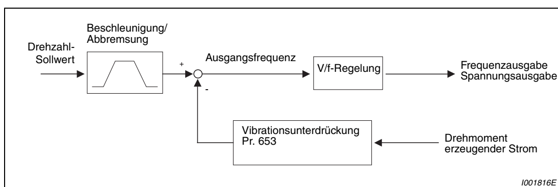
Abb. 6-78: Funktionsweise der Vibrationsunterdrückung
