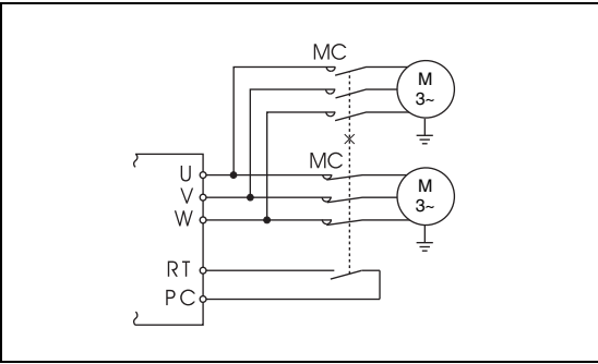
Abb. 6-34: Betrieb von zwei Motoren an einem Frequenzumrichter
