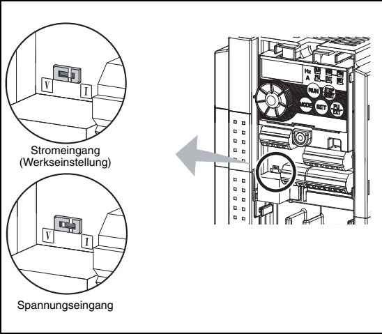
Abb. 6-79: Wahlschalter Spannungs-/Stromeingang
