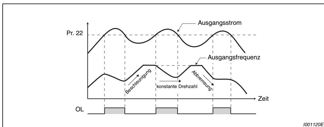
Abb. 6-4: Arbeitsweise der Strombegrenzung
