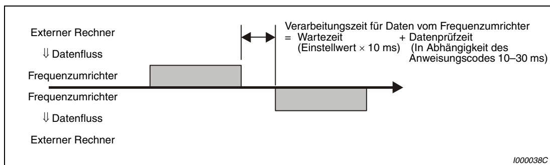
Abb. 6-110: Festlegung der Wartezeit
