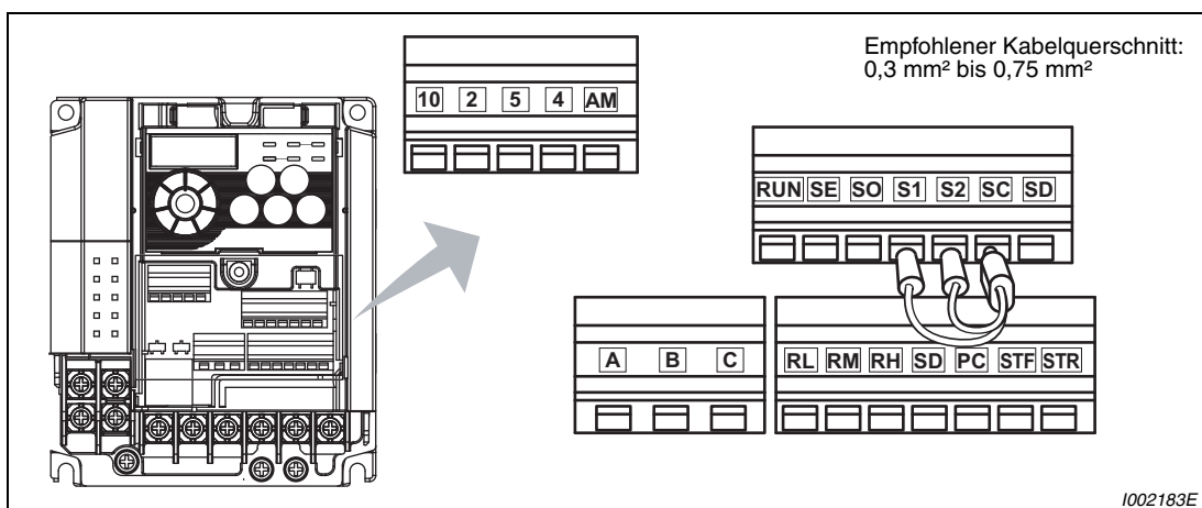
Abb. 3-6: Übersicht der Klemmenbelegung
