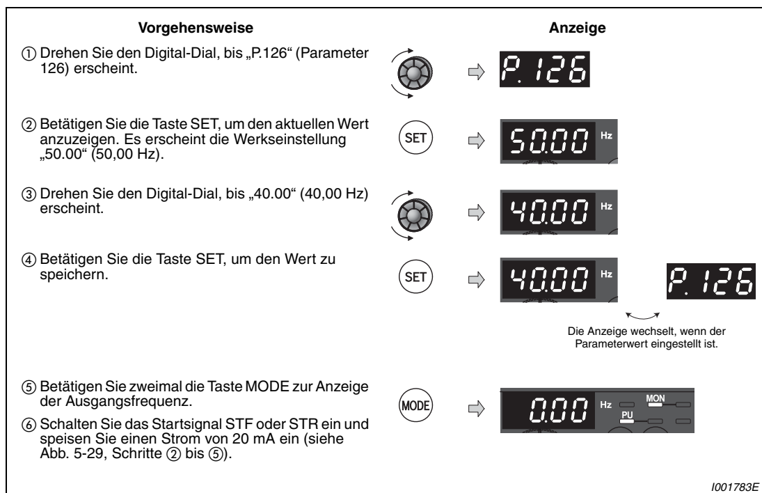
Abb. 5-30: Einstellung der Frequenz bei analogem Maximalwert
