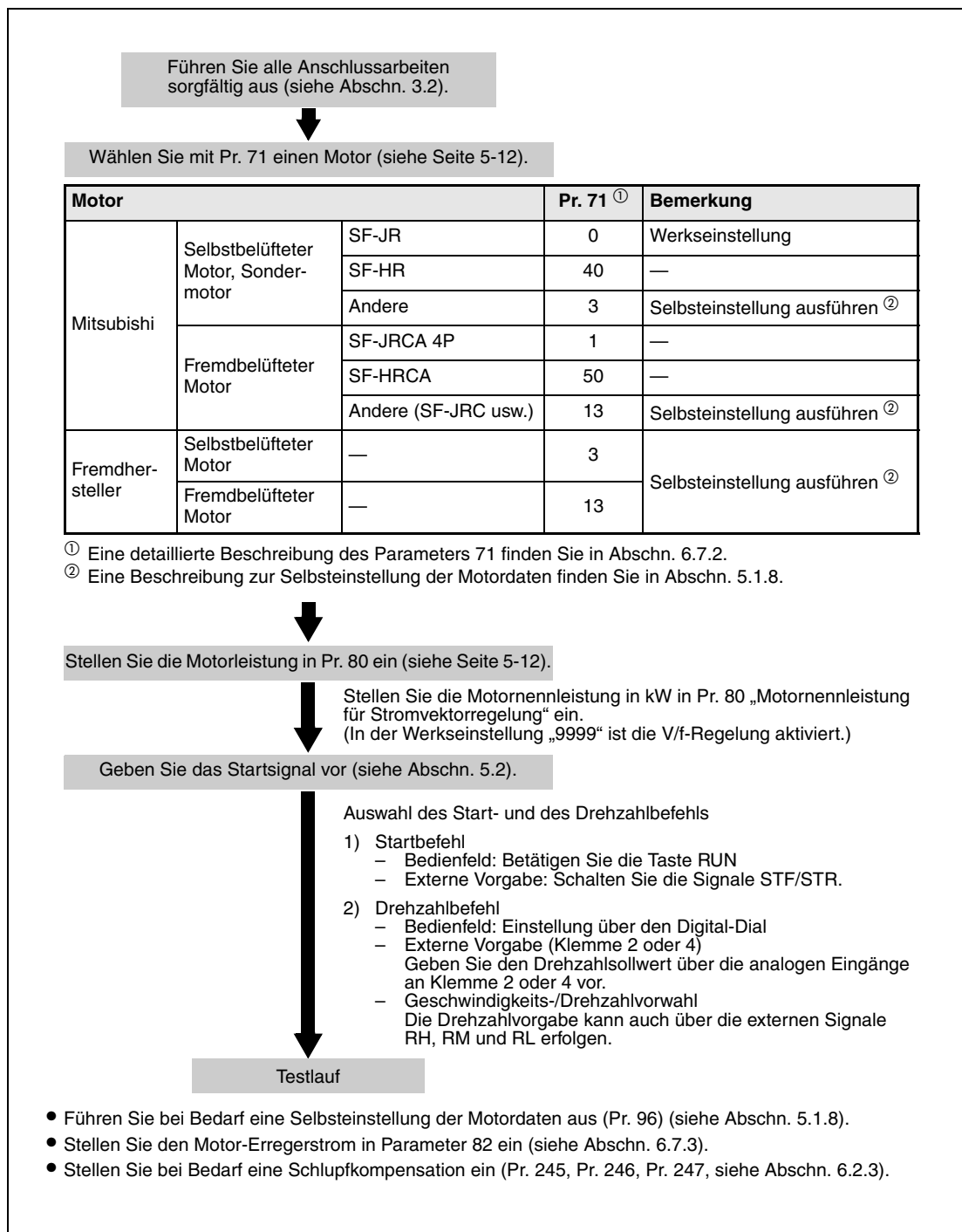
Abb. 5-9: Auswahlmethode der Stromvektorregelung
