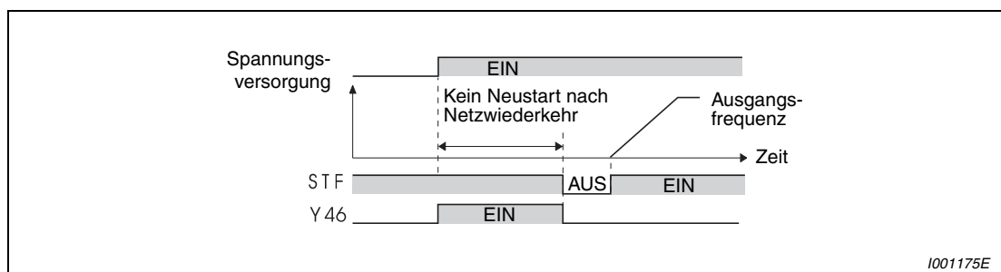
Abb. 6-73: Neustart bei Wiederherstellung der Spannungsversorgung
