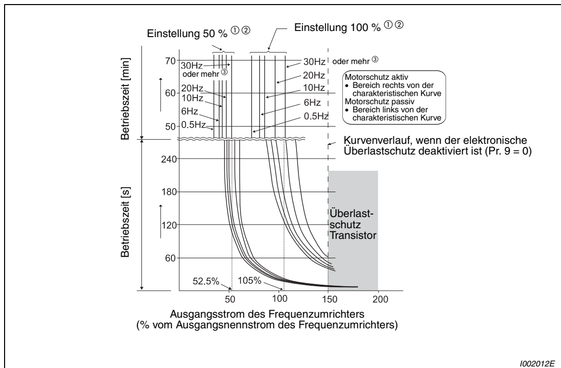
Abb. 6-33: Motorschutz-Kennlinien
