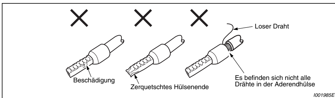
Abb. 3-9: Fehlerhaft verdringte Aderendhülse
