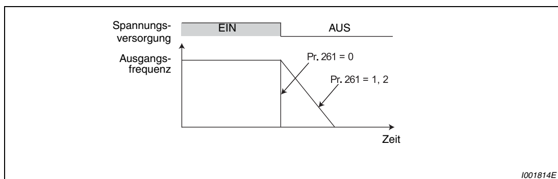
Abb. 6-71: Parameter für Stoppmethode bei Netzausfall
