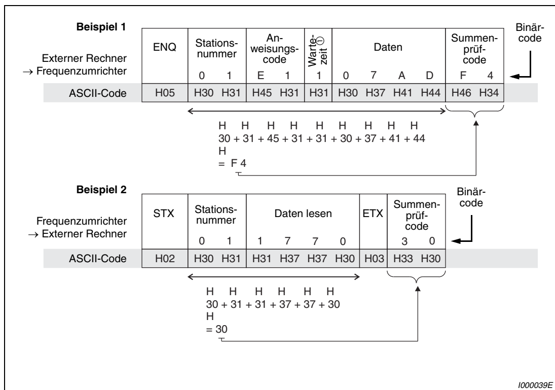
Abb. 6-111: Summenprüfcode (Beispiele)
