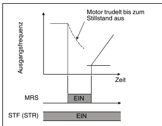
Abb. 6-43: Reglersperre
