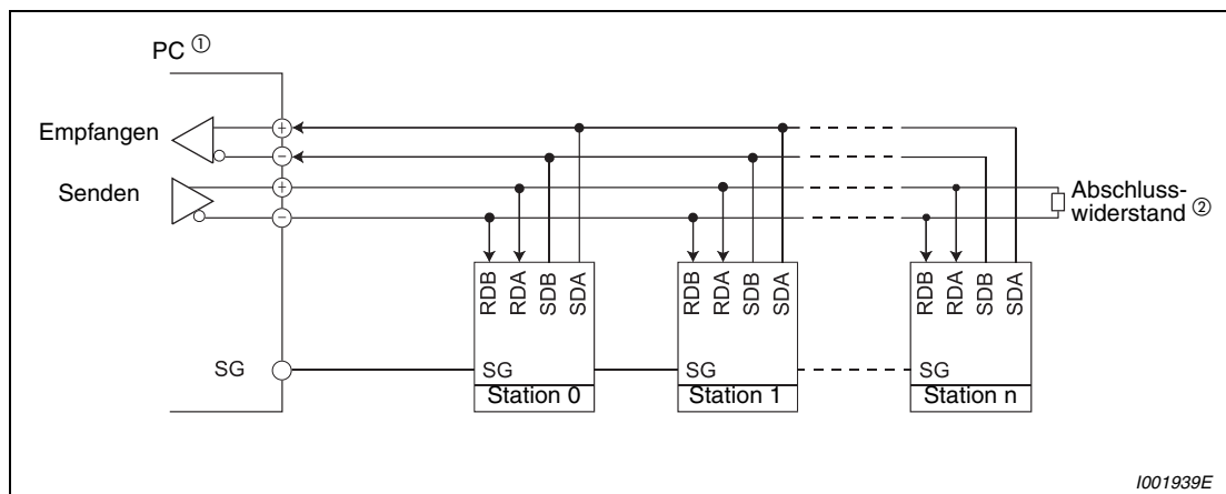
Abb. 6-102: Verkabelung mit mehreren Frequenzumrichtern
