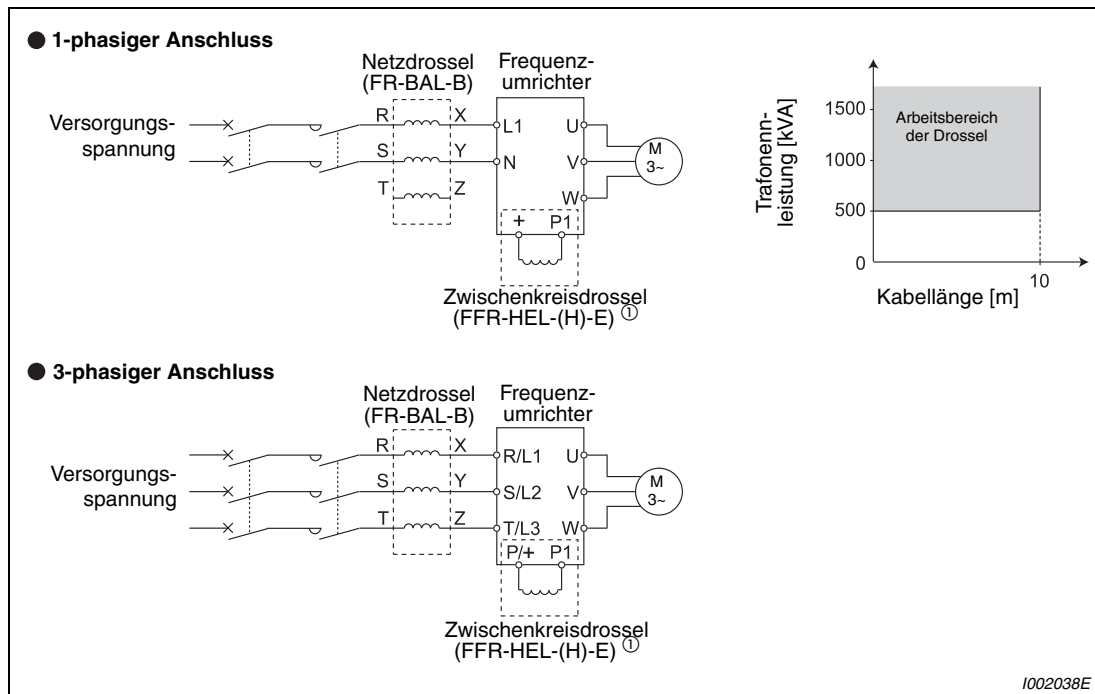
Abb. 3-35: Anschluss einer Netzdrossel
