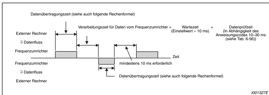
Abb. 6-112: Übertragungszeit
