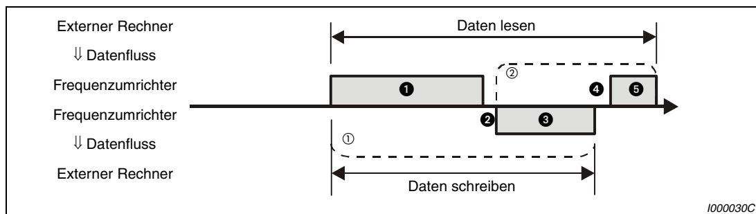
Abb. 6-109: Schematische Darstellung des Datenaustausches
