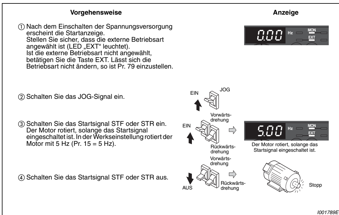
Abb. 6-20: Tipbetrieb in der externen Betriebsart
