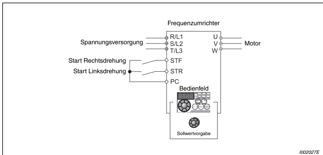
Abb. 5-20: Externe Steuerung
