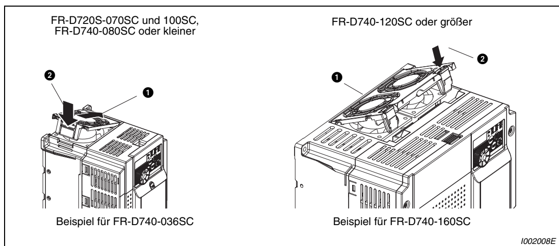
Abb. 8-6: Einbau der Ventilatorabdeckung
