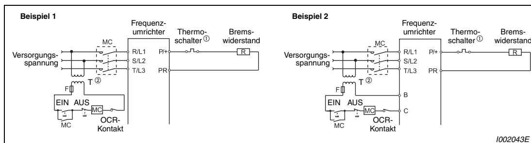
Abb. 3-27: Schutzschaltungen
