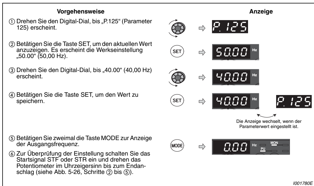
Abb. 5-27: Einstellung der Frequenz für den analogen Maximalwert
