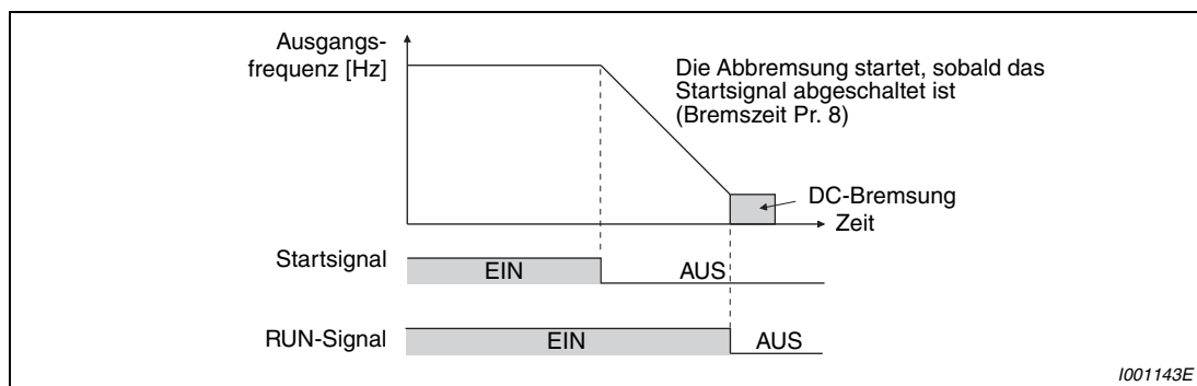
Abb. 6-41: Stoppmethode bei Parameter 250 = 9999
