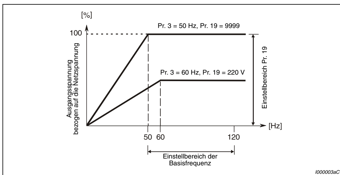
Abb. 6-11: Verhältnis der Ausgangsspannung zur Ausgangsfrequenz
