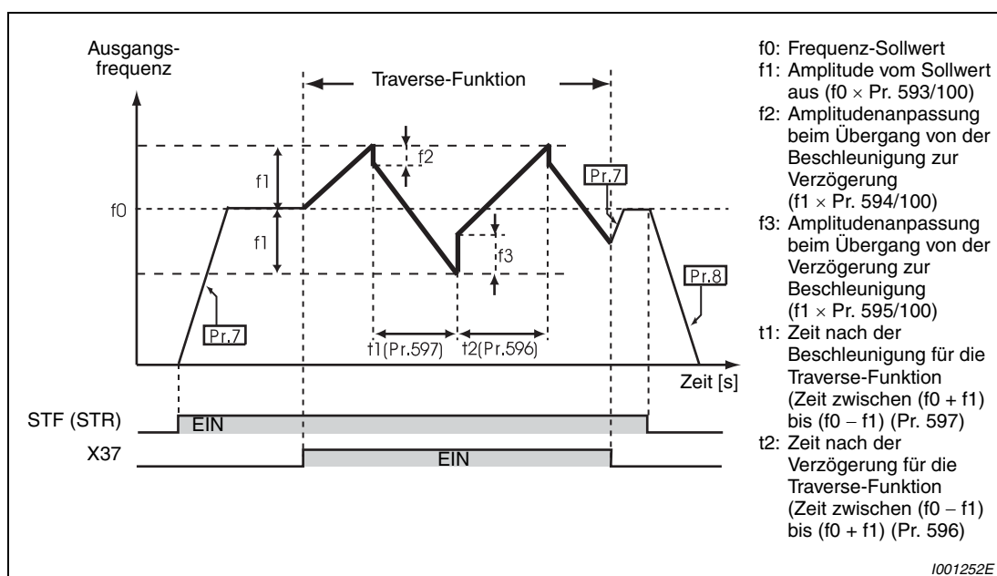
Abb. 6-136: Traverse-Funktion
