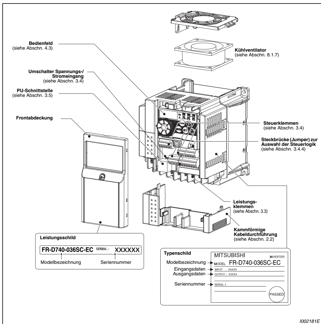
Abb. 1-2: Aufbau des Frequenzumrichters
