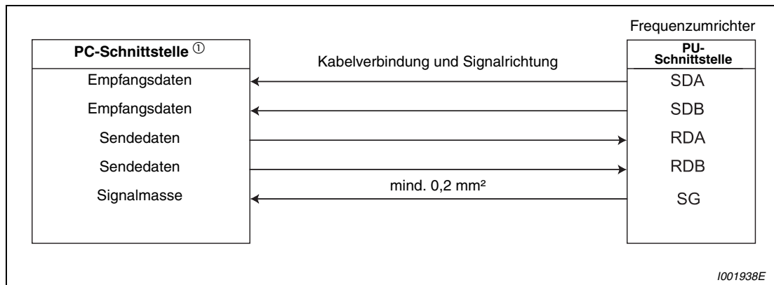
Abb. 6-101: Verkabelung mit einem Frequenzumrichter
