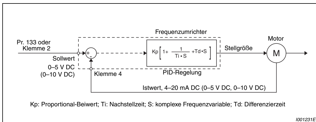
Abb. 6-119: Systemkonfiguration für Pr. 128 = 20 oder 21 (Soll-/Istwertanschluss am Umrichter)
