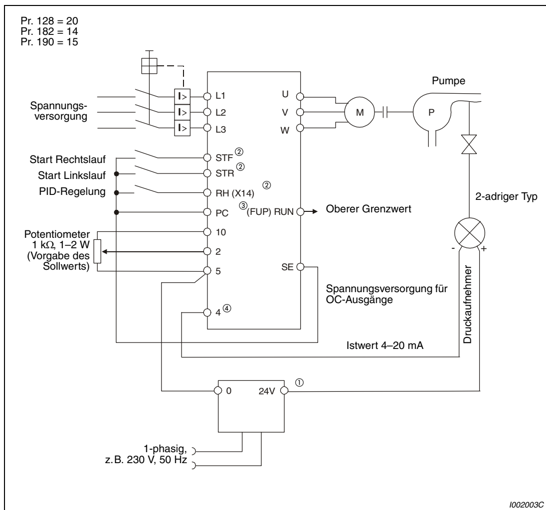
Abb. 6-125: Anschlussbeispiel in positiver Logik
