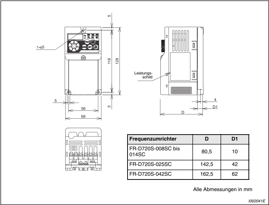
Abb. A-1: Abmessungen der Frequenzumrichter FR-D720S-008SC bis 042SC
