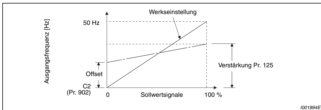
Abb. 6-134: Signalabgleich an Klemme 2
