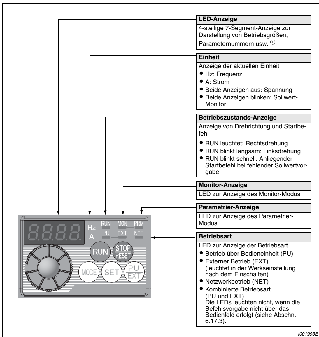
Abb. 4-6: Bedienfeld der Frequenzumrichter der FR-D700 SC
