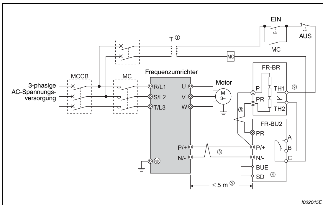
Abb. 3-31: Anschluss der Bremseinheit vom Typ FR-BU2
