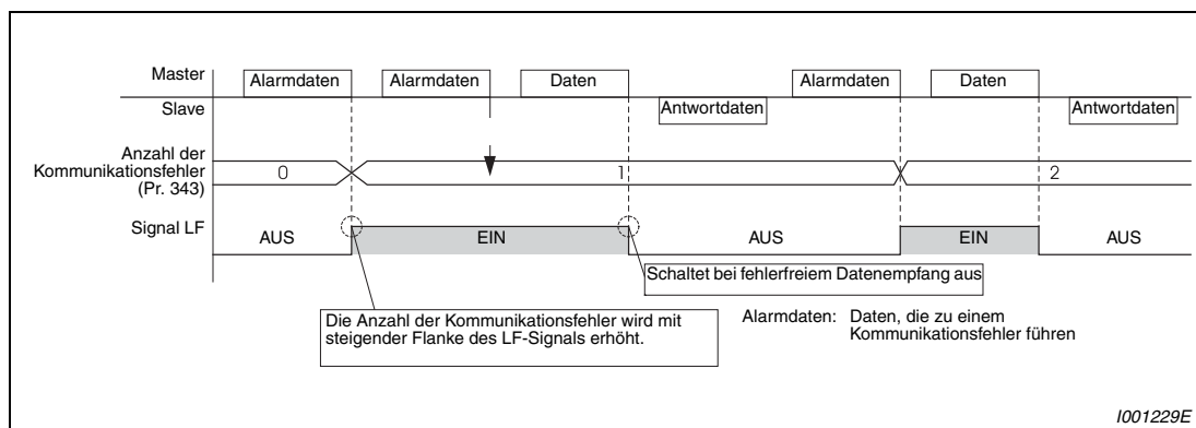
Abb. 6-118: Ausgabe des LF-Signals
