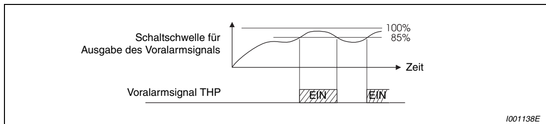
Abb. 6-35: Ausgabe des Voralarmsignals
