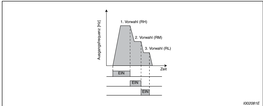
Abb. 6-15: Aufruf der Drehzahlvorwahlen in Abhängigkeit der Signalklemmenbelegung
