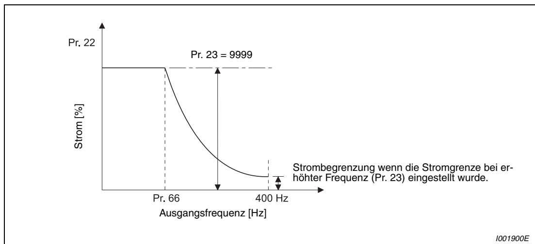
Abb. 6-6: Verlauf der Stromgrenze
