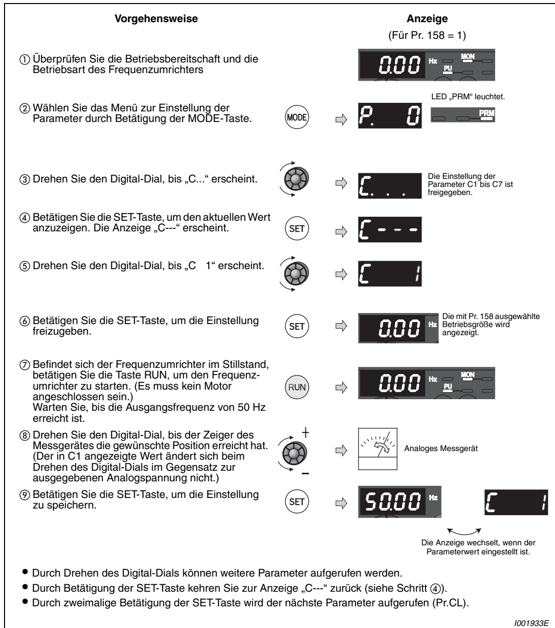
Abb. 6-67: Kalibrierung der AM-Klemme
