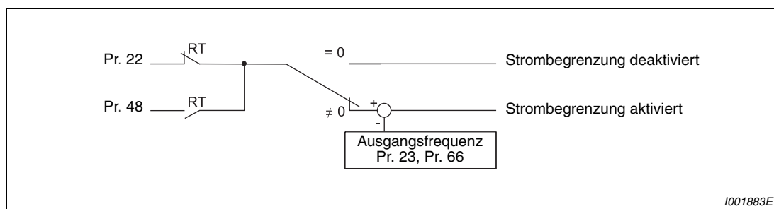
Abb. 6-3: Blockschaltbild der Strombegrenzung
