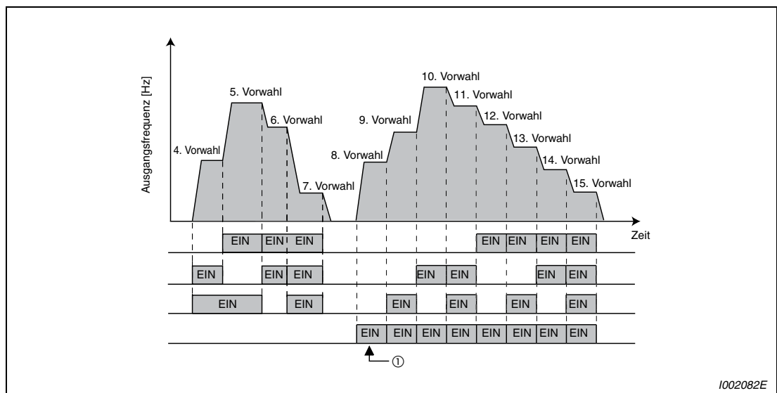
Abb. 6-16: Aufruf der Drehzahlvorwahlen in Abhängigkeit der Signalklemmenbelegung
