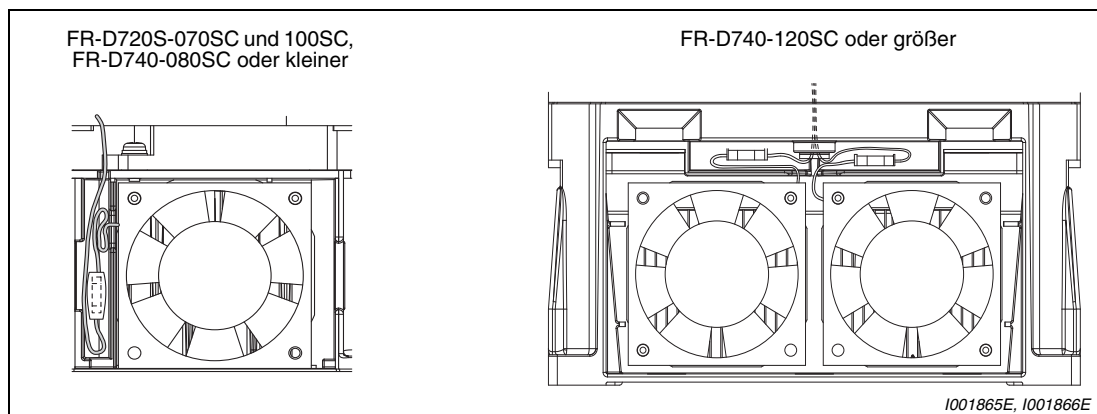
Abb. 8-5: Anschluss des Kühlventilators
