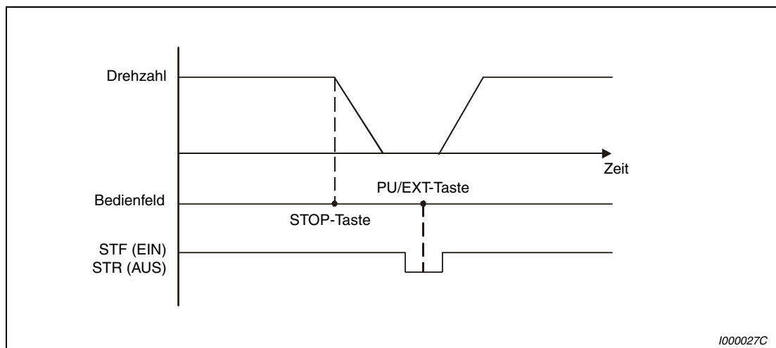
Abb. 6-88: Stopp während der externen Betriebsart
