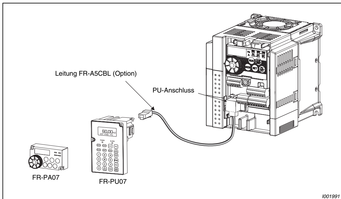
Abb. 3-22: Anschluss einer Bedieneinheit am PU-Anschluss
