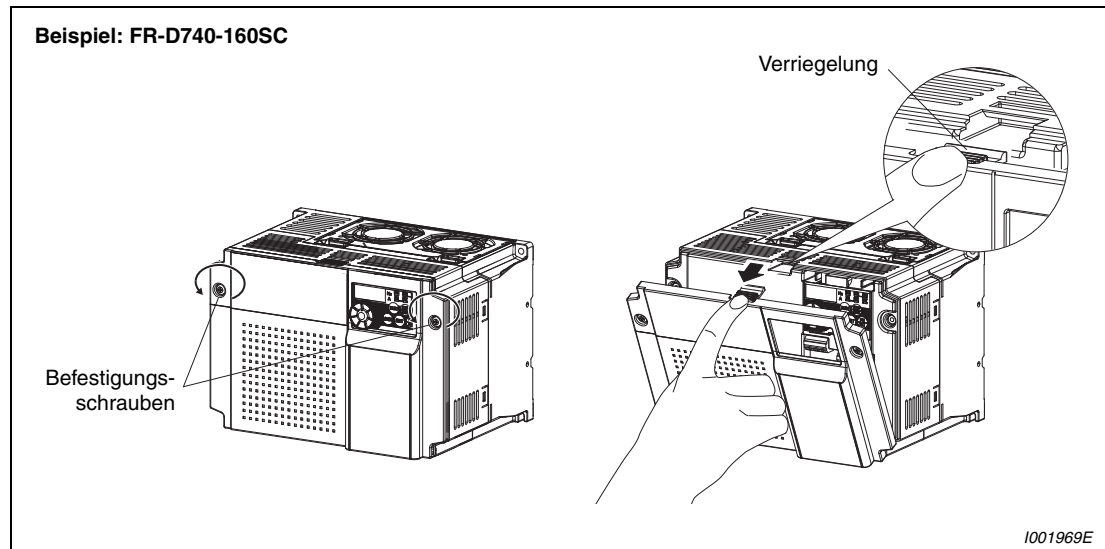
Abb. 2-3: Entfernen der Frontabdeckung
