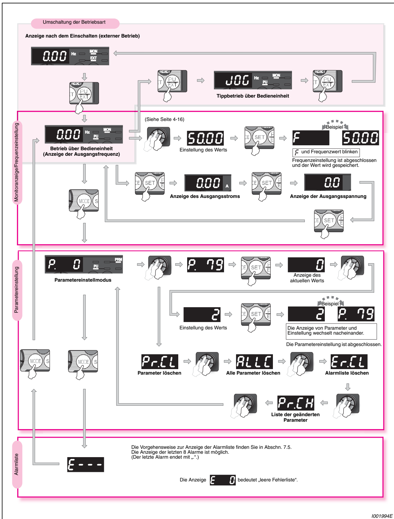
Abb. 4-7: Übersicht der Grundfunktionen des Bedienfeldes
