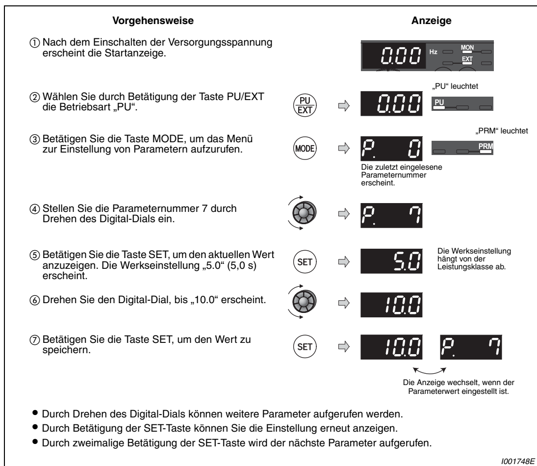
Abb. 5-8: Einstellung der Beschleunigungszeit
