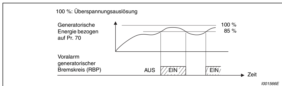
Abb. 6-40: Generatorische Überlast
