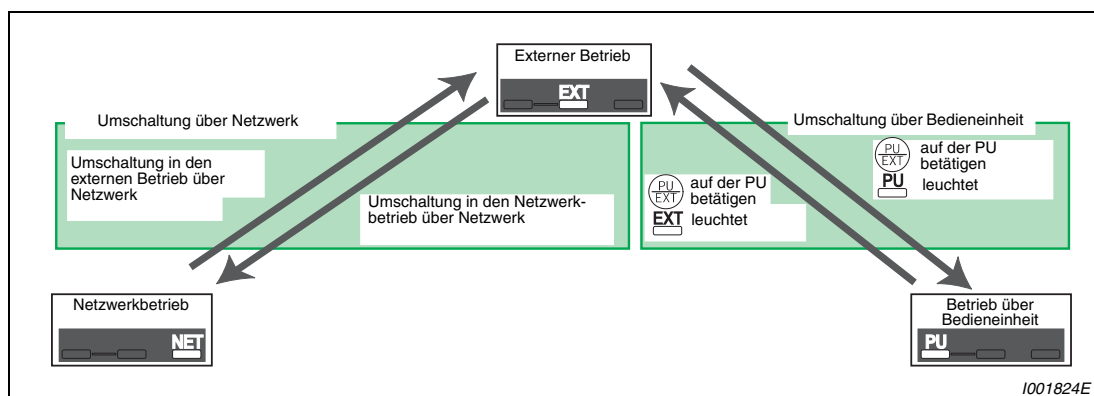
Abb. 6-90: Umschaltung der Betriebsart bei Pr. 340 = 0 oder 1
