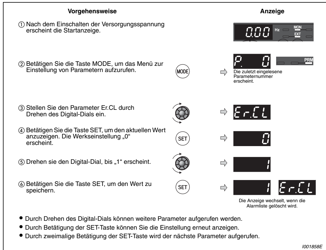
Abb. 7-6: Löschen der Alarmliste
