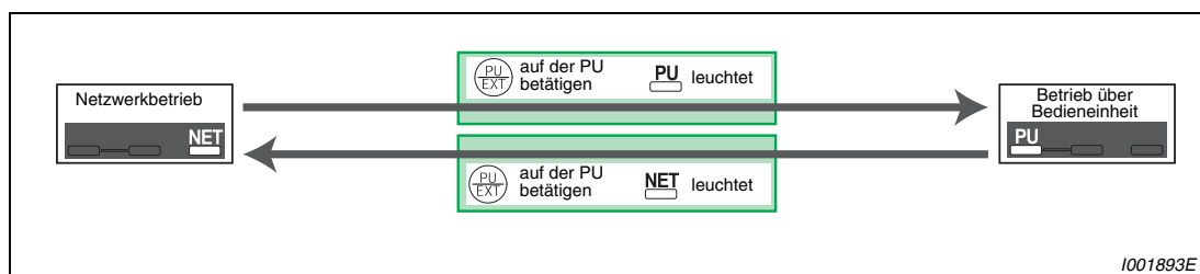
Abb. 6-91: Umschaltung der Betriebsart bei Pr. 340 = 10
