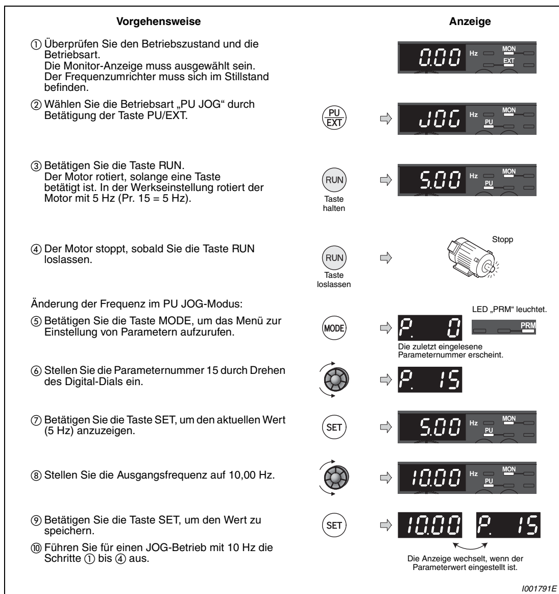
Abb. 6-22: Tippbetrieb über das Bedienfeld
